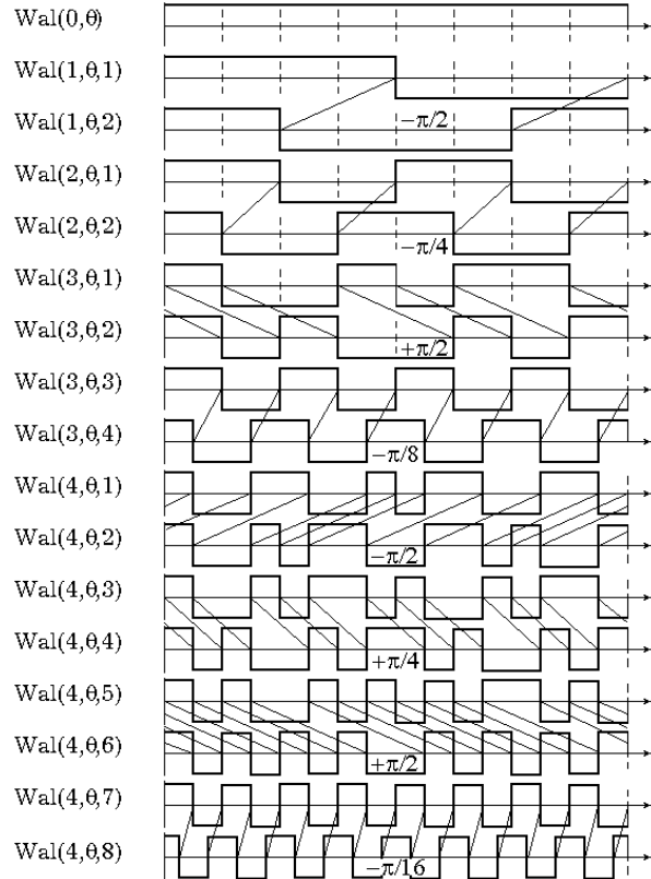
Рис. 2. Фазова взаємозалежність функцій Уолша
