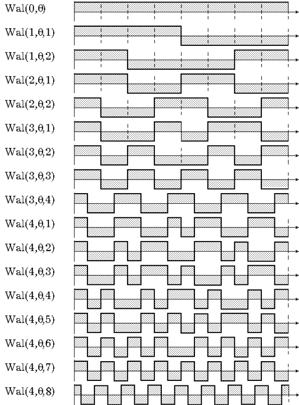
Рис. 1. Функції Уолша, впорядковані за Уолшем
