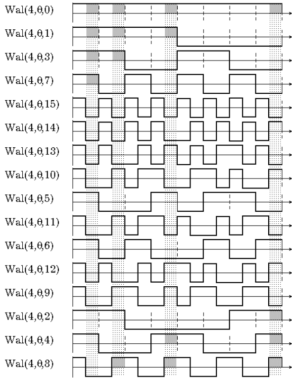
Рис. 3. Базис рекурсивно впорядкованих функцій Уолша
